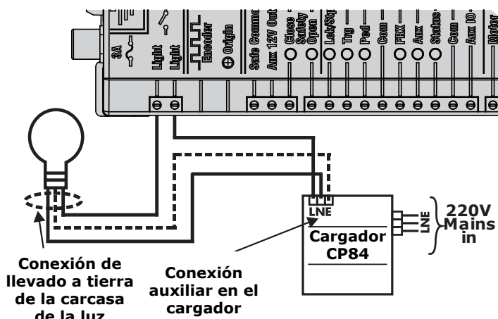
FIGURA 46 CONECCIÓN ESQUEMÁTICA DE LA LUZ
