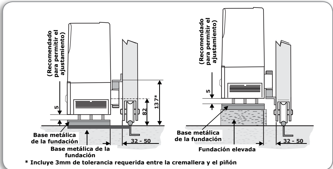
FIGURA 10A CREMALLERA DE NYLON CON SOPORTE DE ACERO ANGULADO, SOBRE EL PIÑÓN
