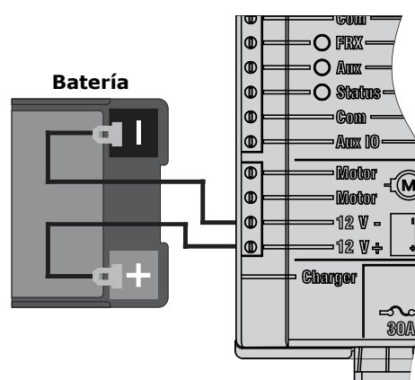
FIGURA 45 CONECCIÓN ESQUEMÁTICA DE LA BATERÍA
