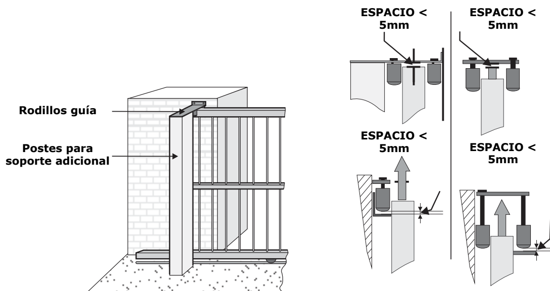
FIGURA 4 MONTANDO LOS RODILLOS GUÍAS
